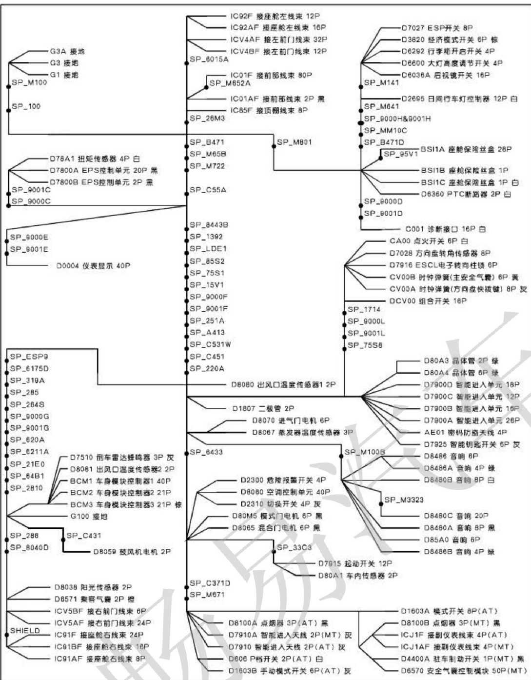
仪表板线束结构图
